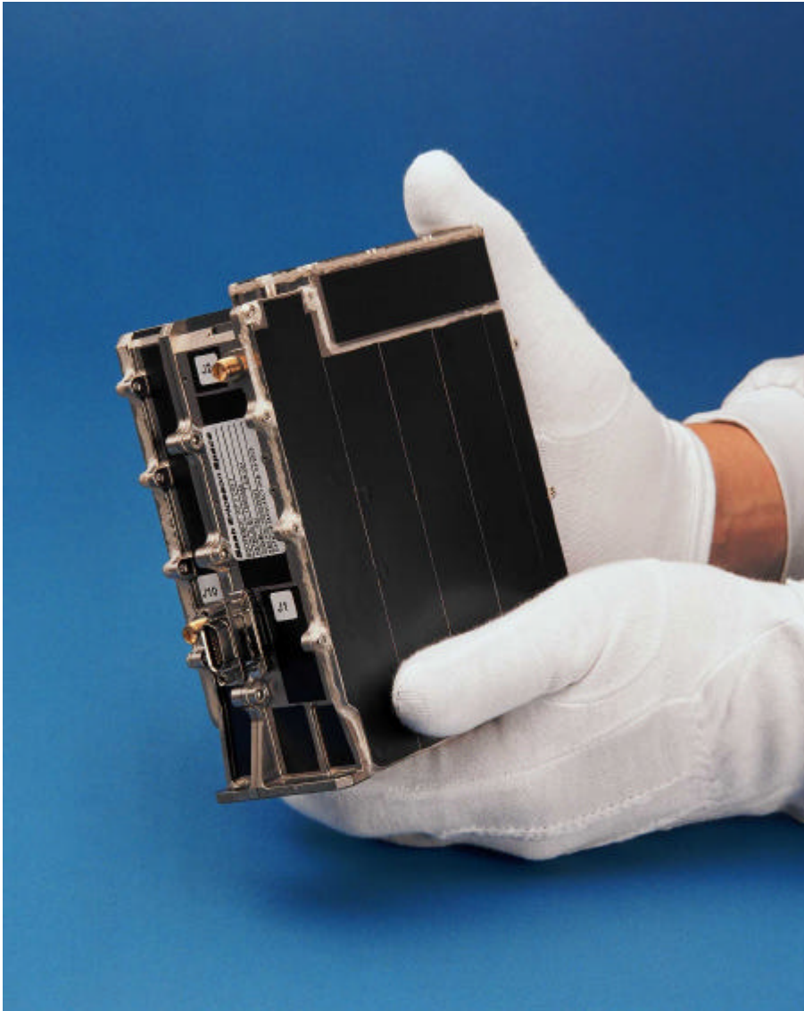
Frekvensomvandlare av den typ som nu beställts för JCSAT-10.
