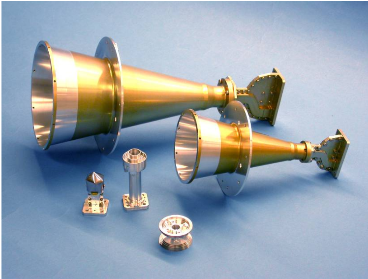
DIRECTV familj av bredtäckande antenner under tillverkning.
